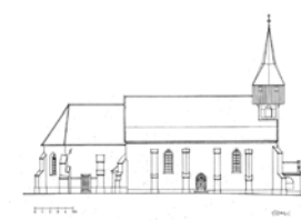
Az északi homlokzat felmérési rajza
