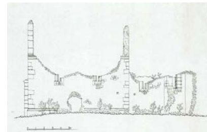
A déli homlokzat felmérési rajza
