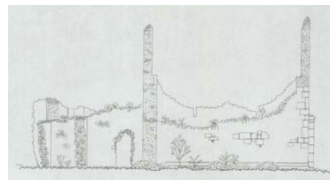
Az északi homlokzat felmérési rajza
