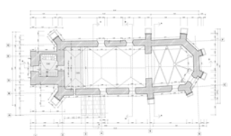
A templom karzatszinti alaprajza
