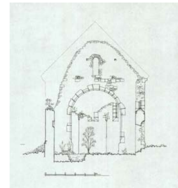
A romtemplom keresztmetsete
