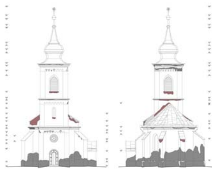
A nyugati és keleti homlokzat felmérési rajza
