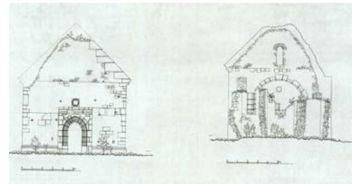
A nyugati és keleti homlokzat felmérési rajza
