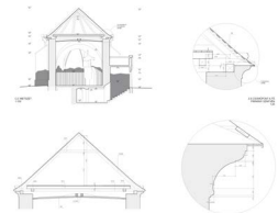
A fedélszék metszete és a főpárkány profilja
