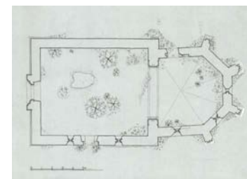
A romtemplom alaprajza
