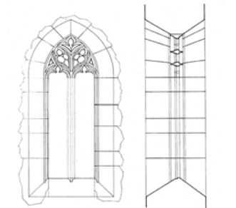
A szentélyablak felmérési rajza
