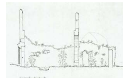
A romtemplom hosszmetsete
